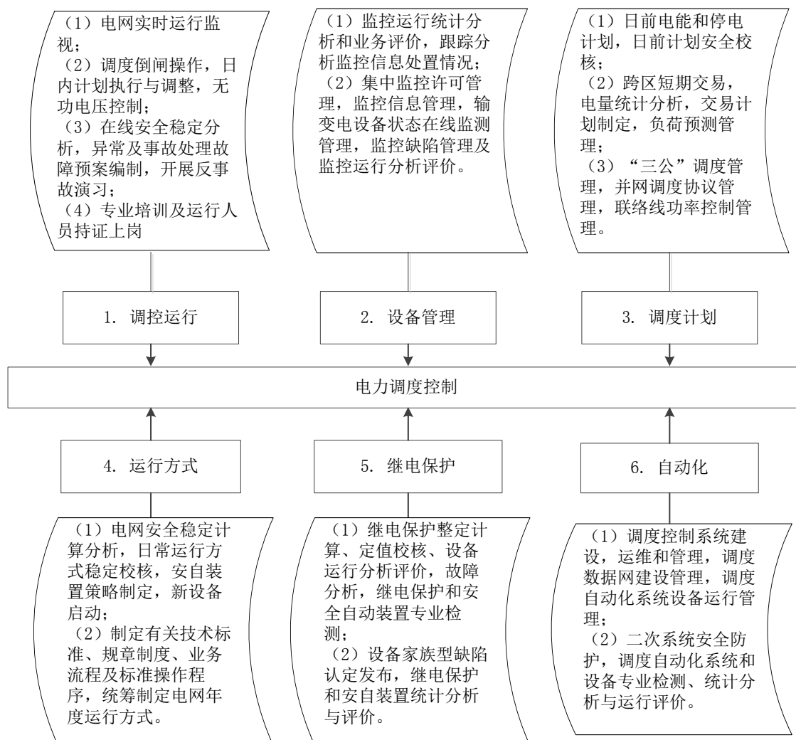
图 5-5 调度控制业务流程
